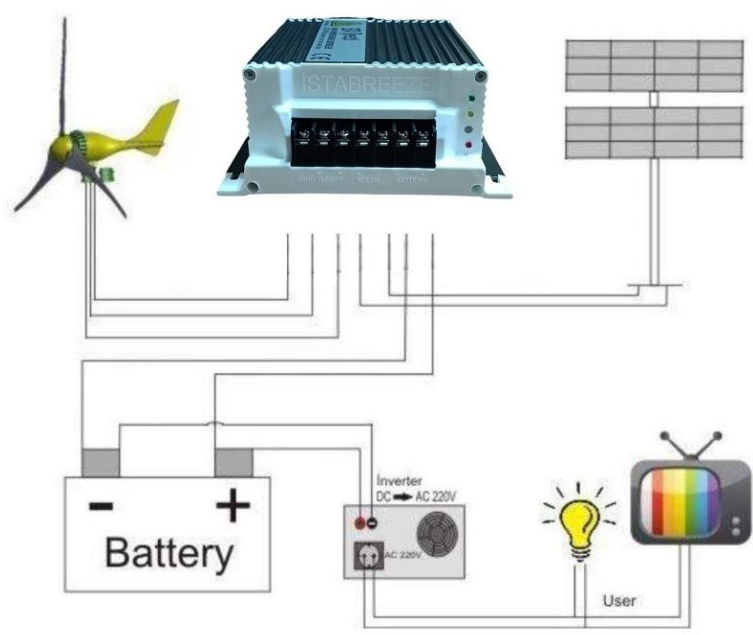
Schaltplan Beispiel
