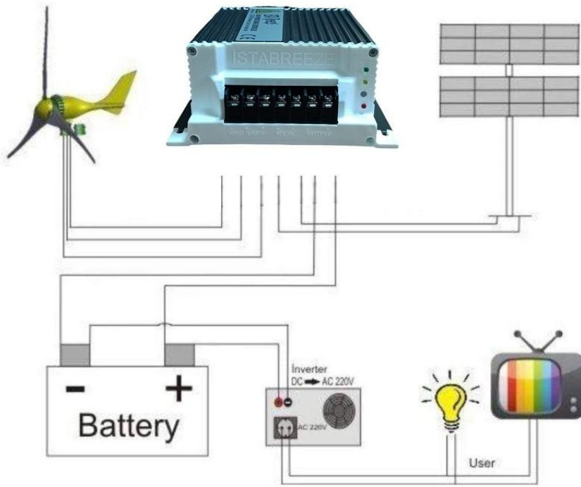
Örnek bağlantı şeması
